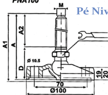
DIMENSÕES PNA100
