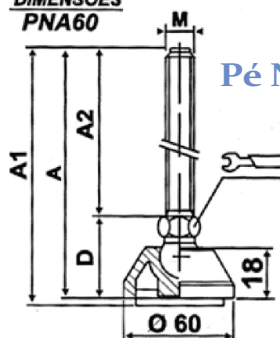
DIMENSÕES PNA60
